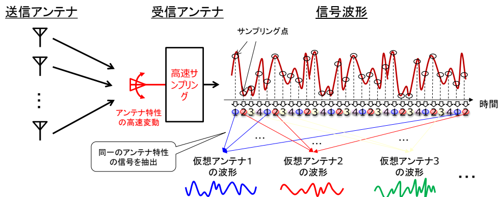
図 4-9. 周波数帯域幅よりも大きいサンプリングレートをを用いる非直交伝送技術の例 (VM-MIMO)
