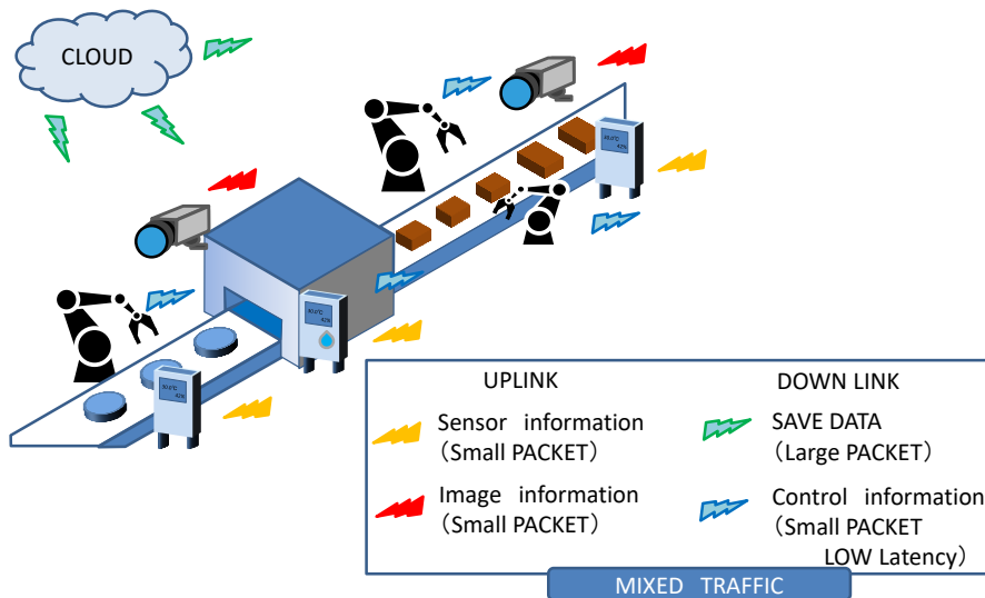
図 4-10. 産業向けネットワークにおける様々なトラフィックのサポート
