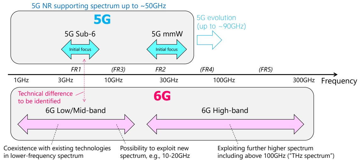
図 4-6. 6G に向けた周波数帯の開拓
