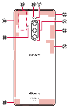
背面
